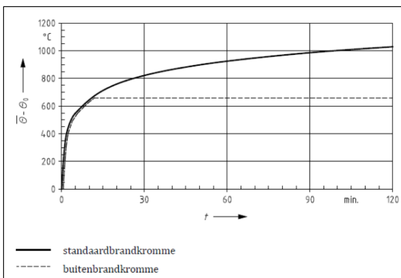
Afb. 4.2: Standaardbrandkromme en buitenbrandkromme [NEN 6069]
