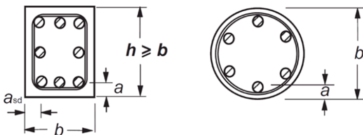
Afb. A.3: Schematische weergave van de betondekking op de wapening.
