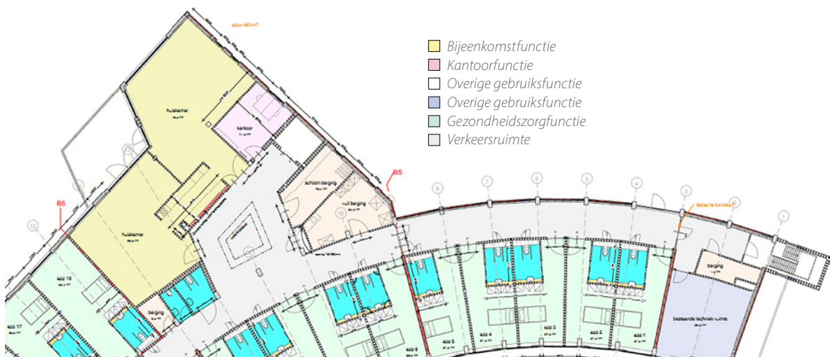
Afb. 1.1: Plattegrondtekening met indeling in gebruiksfuncties
