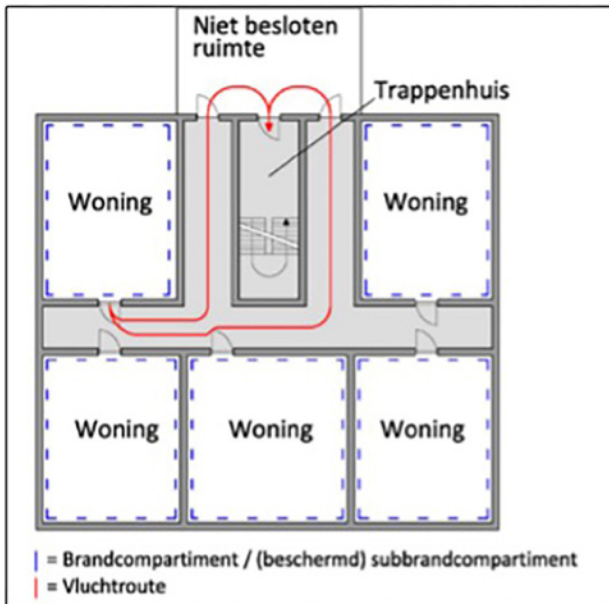
Afb. 2.3: Via niet besloten ruimten: veiligheidsvluchtroute
