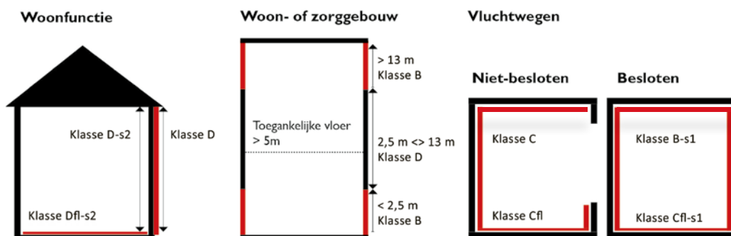
Afb. 3.1: Wanneer welke brandklasse-eis?
