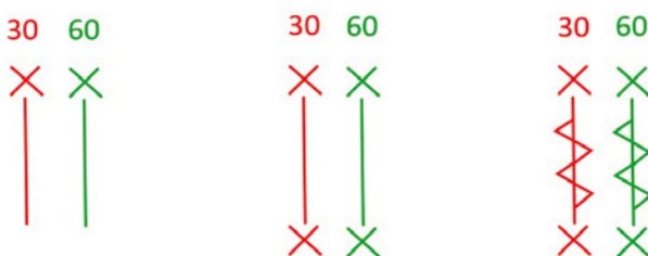
Afb. 1.4: De kleur en het cijfer geven de hoogte van de brandwerendheid aan. [bron: NEN 1413]
