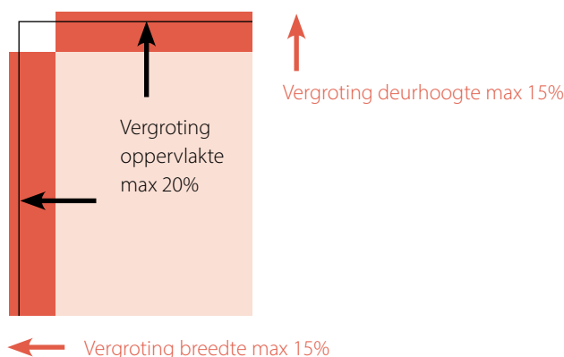
Afb. E.2: Maximaal toegestane vergrotingen van de deurafmetingen.
