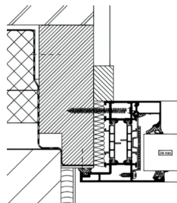
Afb. G.3: Typisch Nederlandse aansluiting van een brandwerende aluminium pui (vast glas) in een houten stelkozijn.
