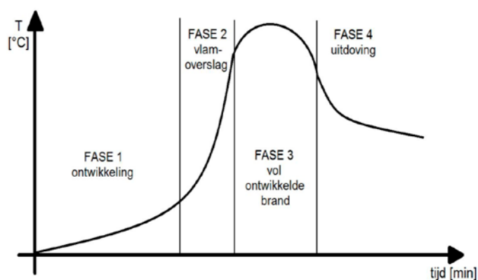
Afb. 6.3: Fasen in de ontwikkeling van een brand
