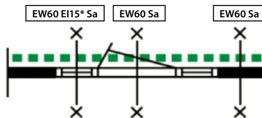
Afb. 1.7: Weergave eisen brandwerendheid en rookdoorlatendheid puiconstructie [bron NEN 1413]
