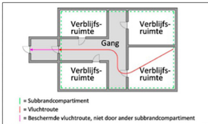
Afb. 2.1: Buiten subbrandcompartiment (maar binnen brandcompartiment): beschermde vluchtroute
