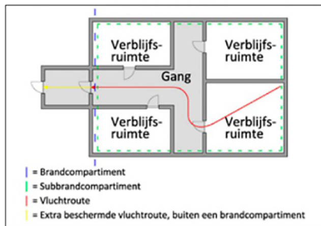
Afb. 2.2: Buiten brandcompartiment: extra beschermde vluchtroute
