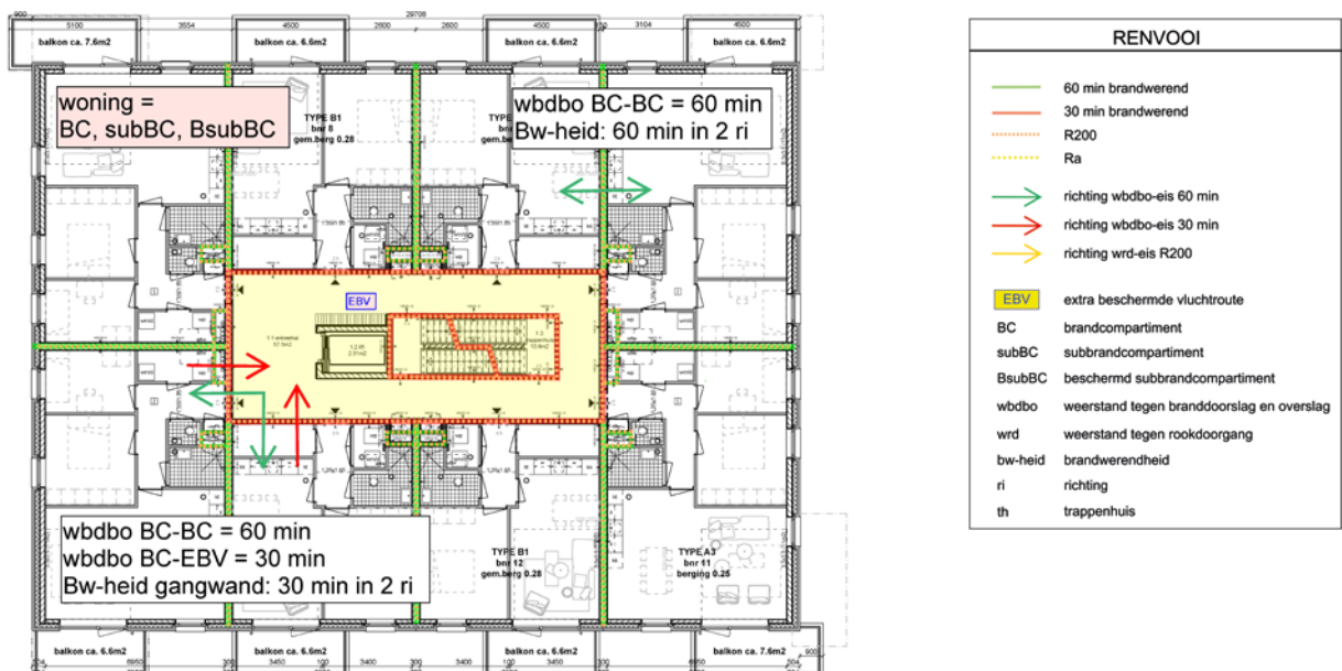
Afb. 3.3: Woongebouw: van wdbbo-eis naar eis brandwerendheid
