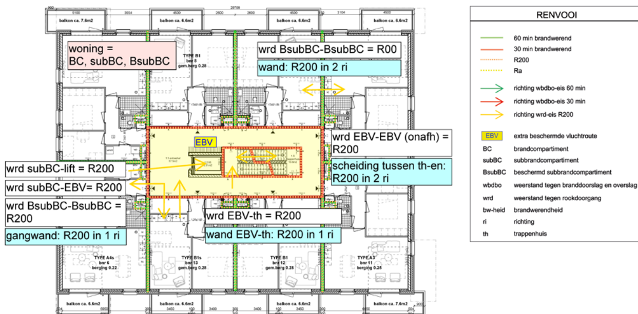
Afb. 3.4: Woongebouw: van wrđ-eis naar eis rookwerendheid
