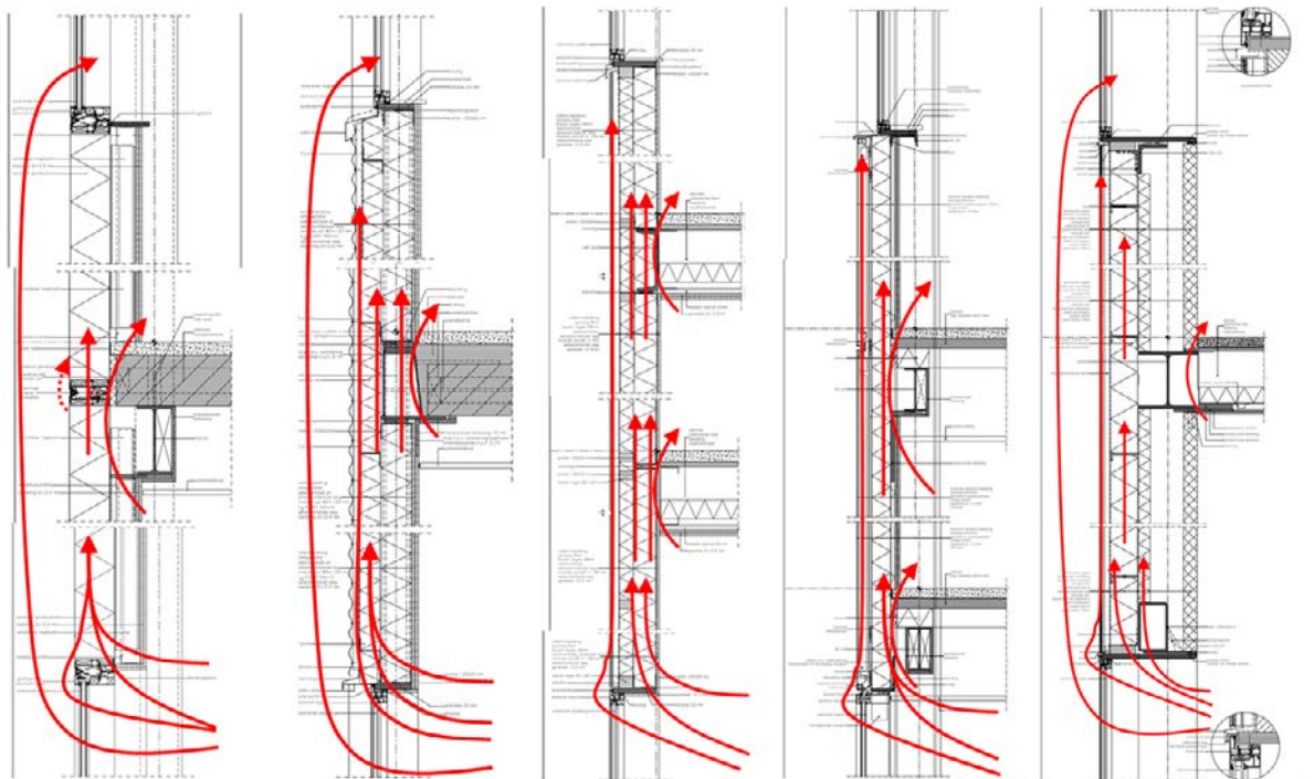
Figuur 12: Alle branddoorslag- en brandoverslagtrajecten moeten worden beschouwd in de bepaling van de aanwezige wbdbo
