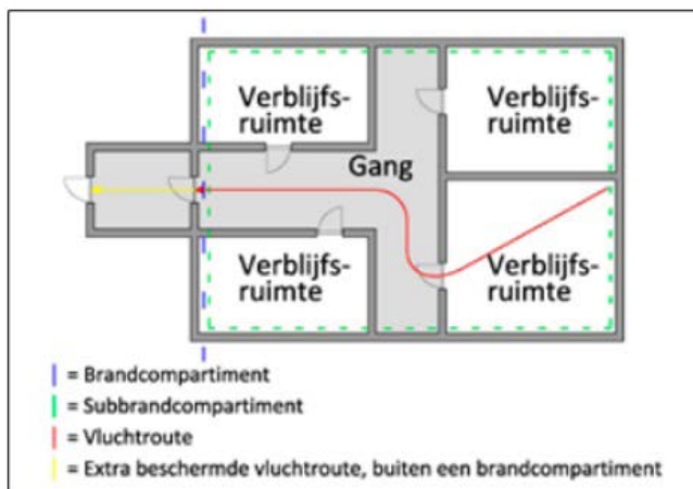
Figuur 9: Buiten brandcompartiment: extra beschermde vluchtroute
