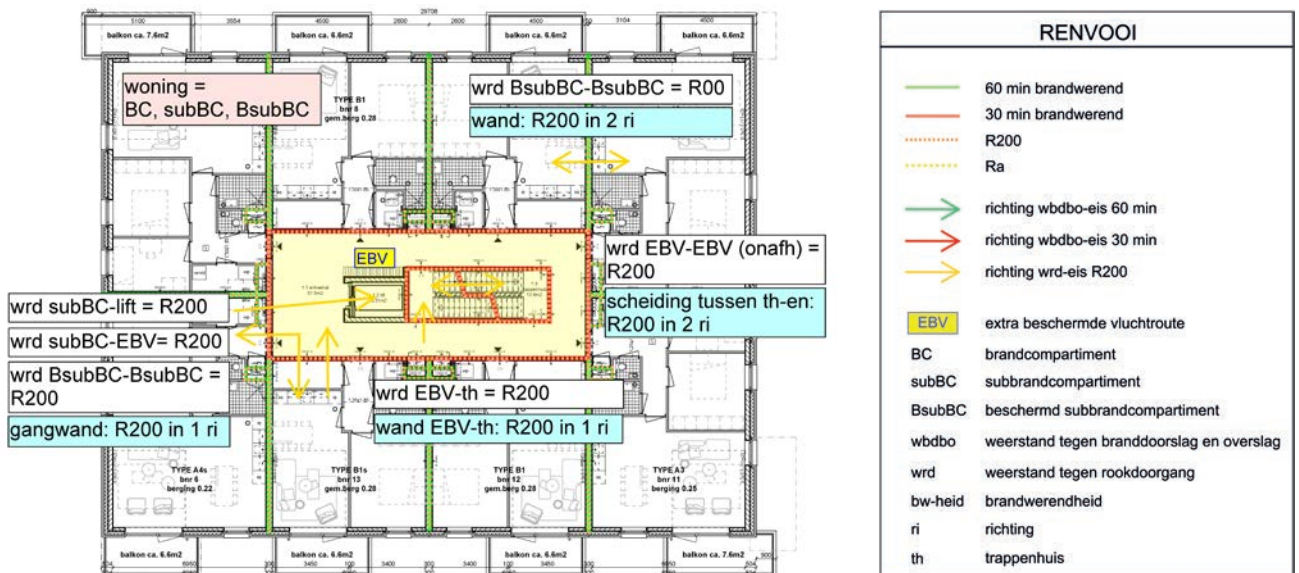
Figuur 14: Woongebouw: van wrd-eis naar eis rookwerendheid
