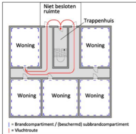
Figuur 10: Via niet besloten ruimten: veiligheidsvluchtroute
