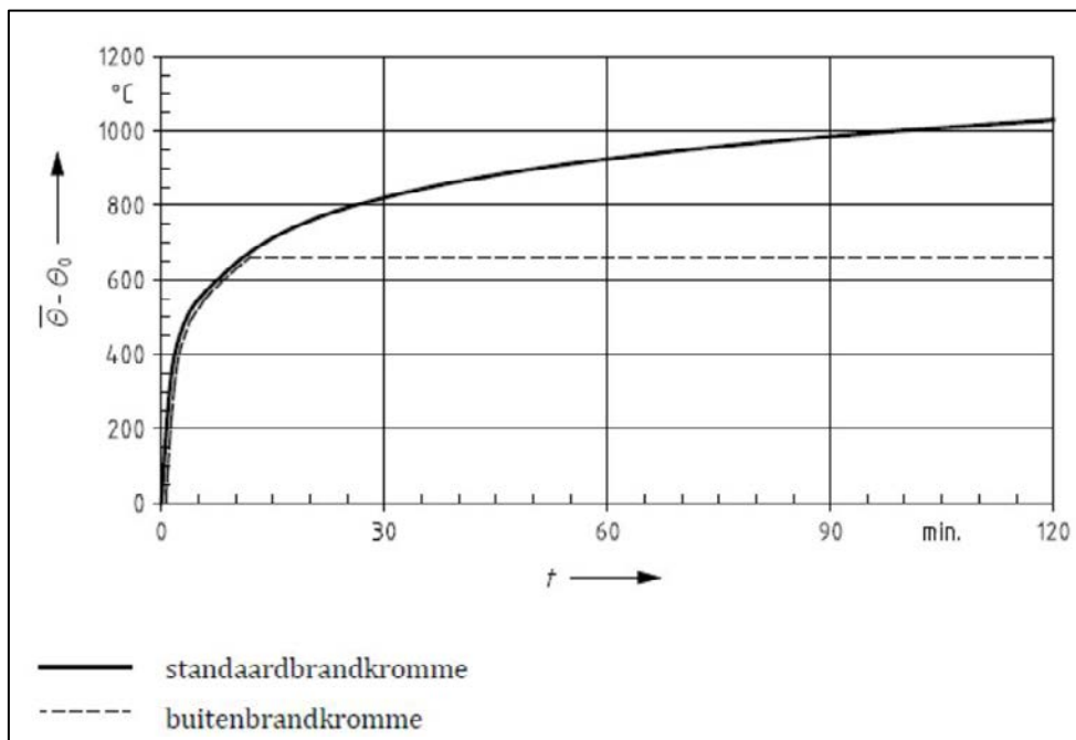
Figuur 15: Standaardbrandkromme en buitenbrandkromme [NEN 6069]
