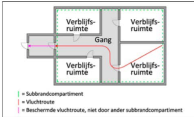
Figuur 8: Buiten subbrandcompartiment (maar binnen brandcompartiment): beschermde vluchtroute
