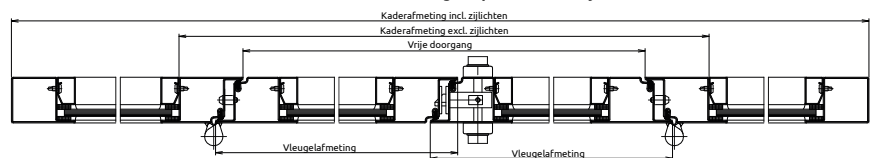
Doorsnede aanslagdeur/wisseldeur + zijlichten
